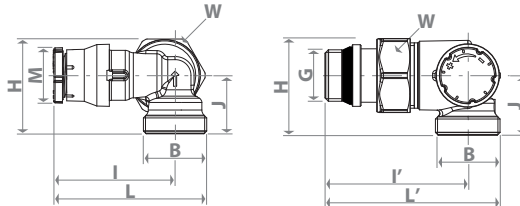
CONEXIÓN ADAPTADOR
